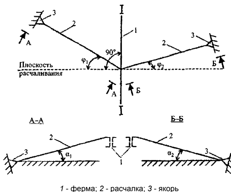
Рисунок К.2 - Схема раскрепления ферм расчалками
