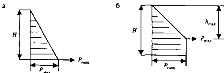
Рисунок Г.1 — Расчетные эпюры бокового давления бетонной смеси
